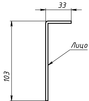
Схема сгиба
