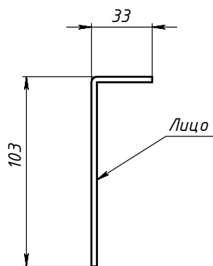
Схемагиба
