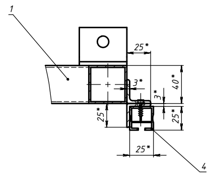
H-H (1 : 2)
