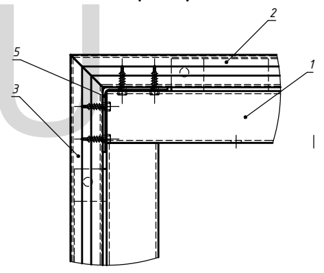
J (1 : 2)
